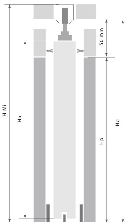
SECCIÓN VERTICAL seção vertical
