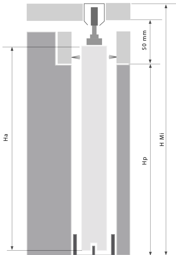
SECCIÓN VERTICAL seção vertical
