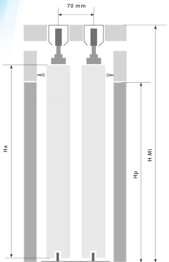
SECCIÓN VERTICAL seção vertical
