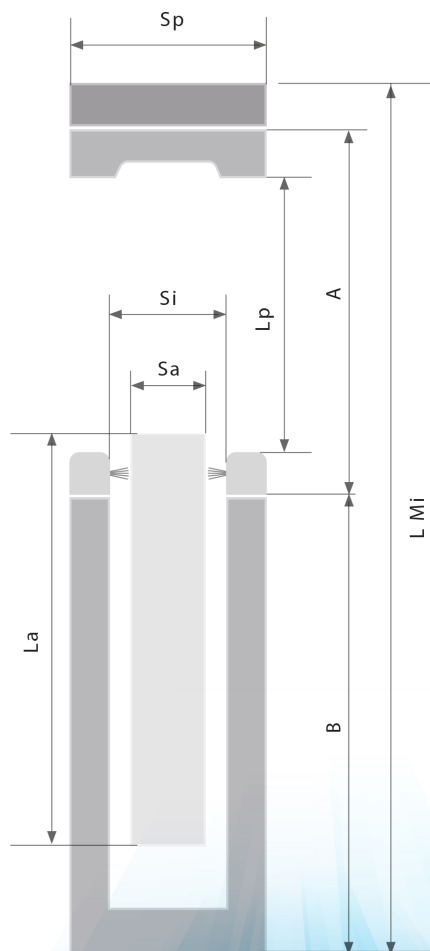
SECCIÓN HORIZONTAL seção horizontal
